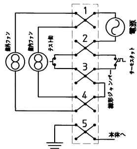
結線図
